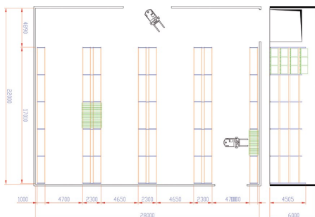
Capacité initiale : 480 palettes (dimensions palettes : 1000 x 1200 mm)
