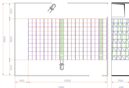
Nouvelle capacité : 800 palettes (dimensions palettes 1000 x 1200 mm)
