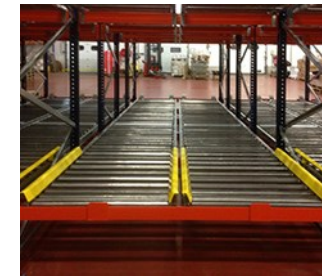
Guides de dépose et protecteur de rouleaux
