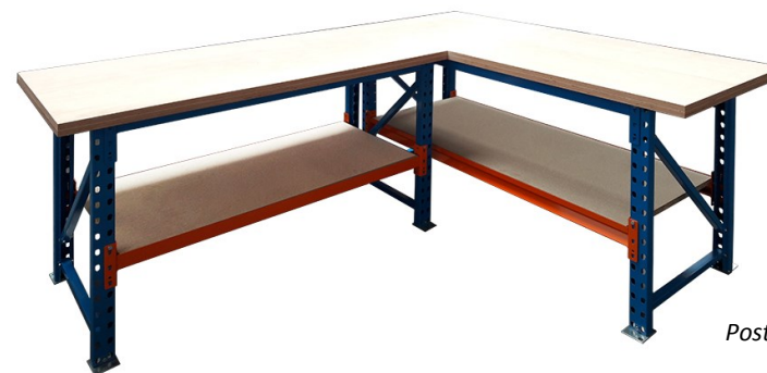
Plateau aggloméré, repose-pieds
